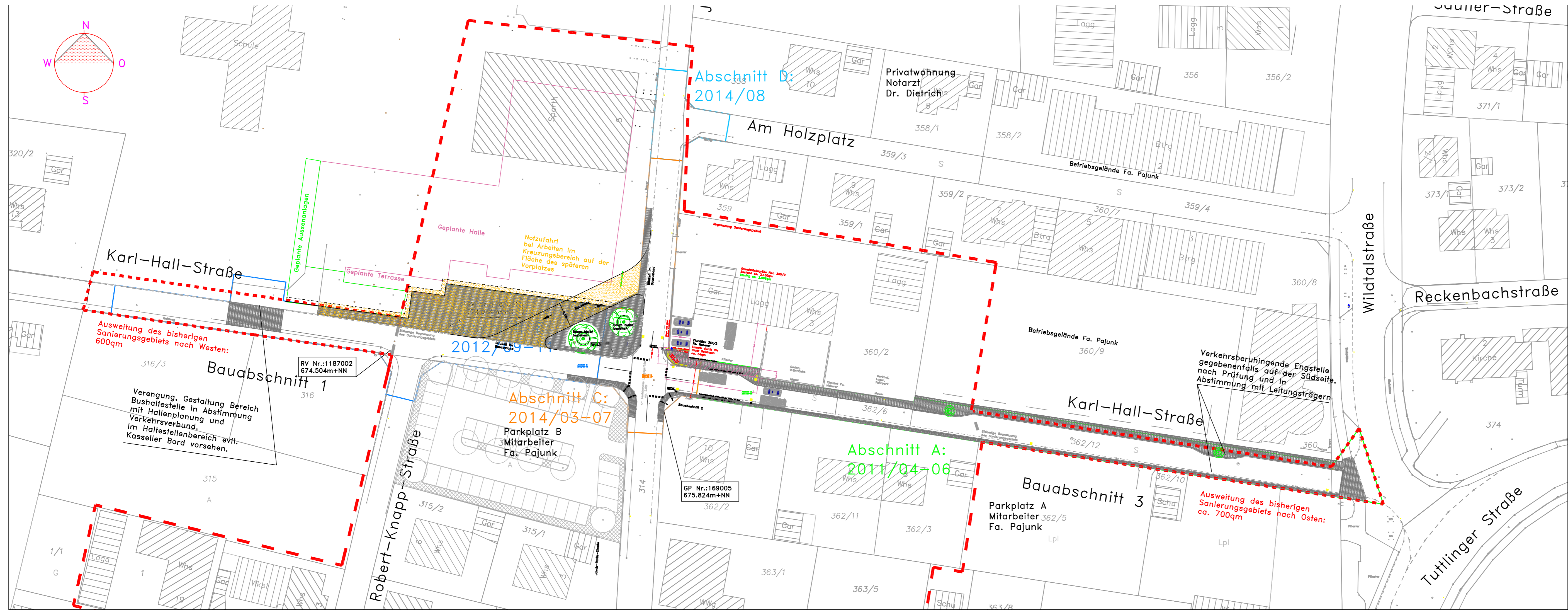
Zeichnung : Lageplan M = 1:500
