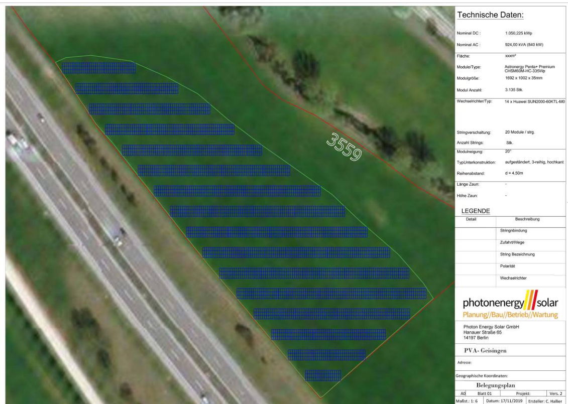
Abb. 3: Belegungsplan der PVA (solarcomplex 17.11.2019)
